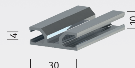
AL 30-10 2004-0110
