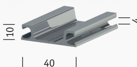
AL 40-10 2005-0040
