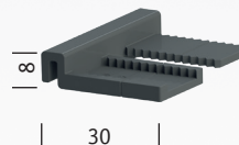
Verbindungselement Connection element 103 225
