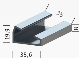
AL 35-14 W 2003-0100
